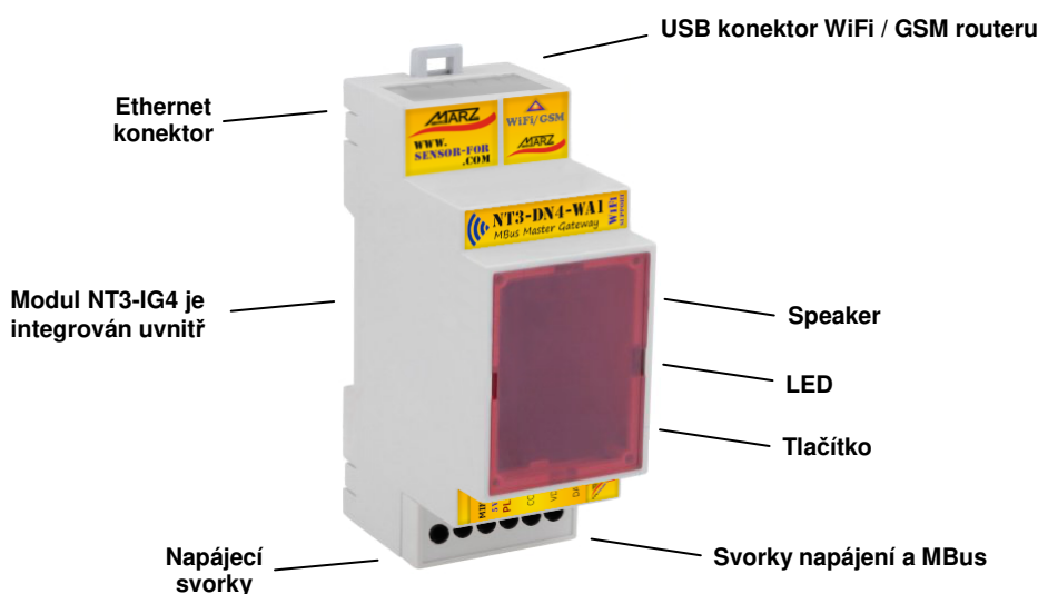
Obr. 2 NT3-DN4-WA1, popis zadní a přední strany
